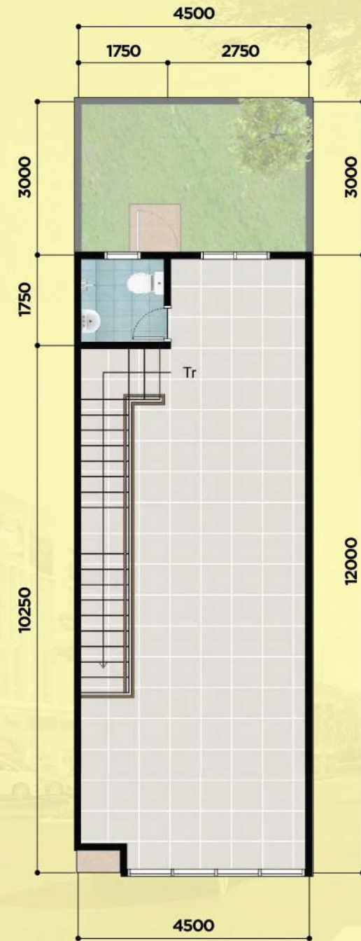
Lantai 3
