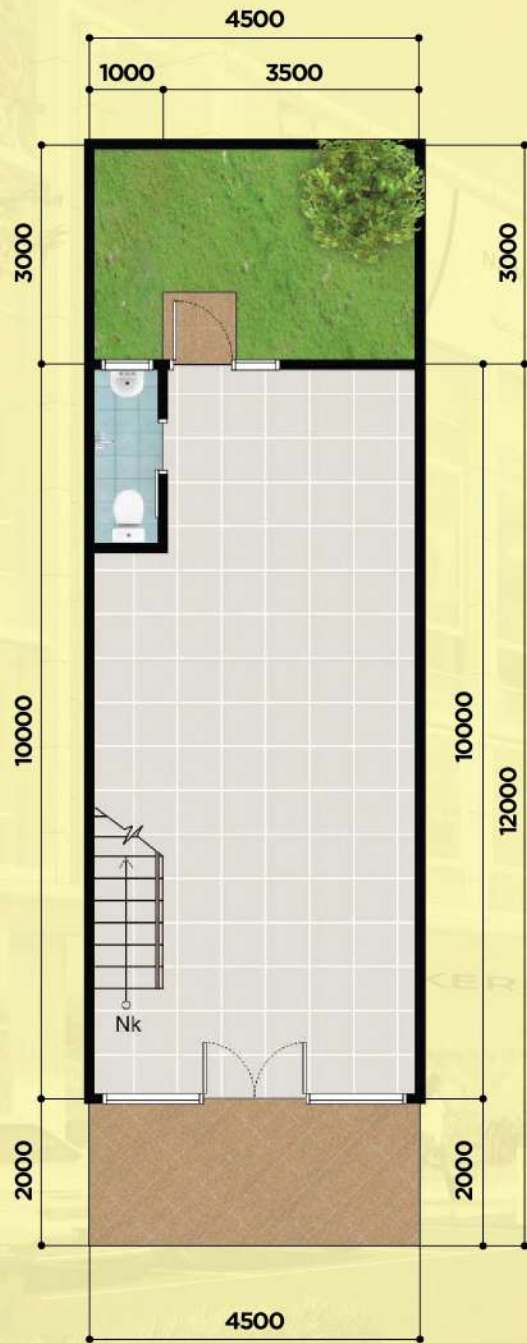
Lantai Dasar
