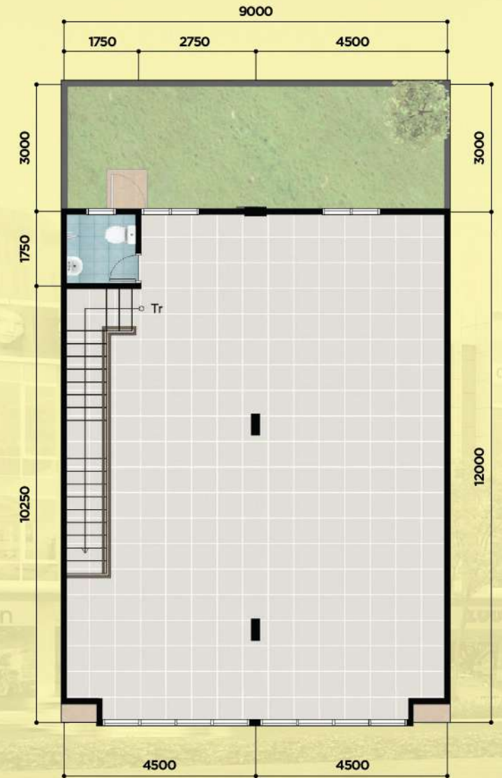
Lantai 3
