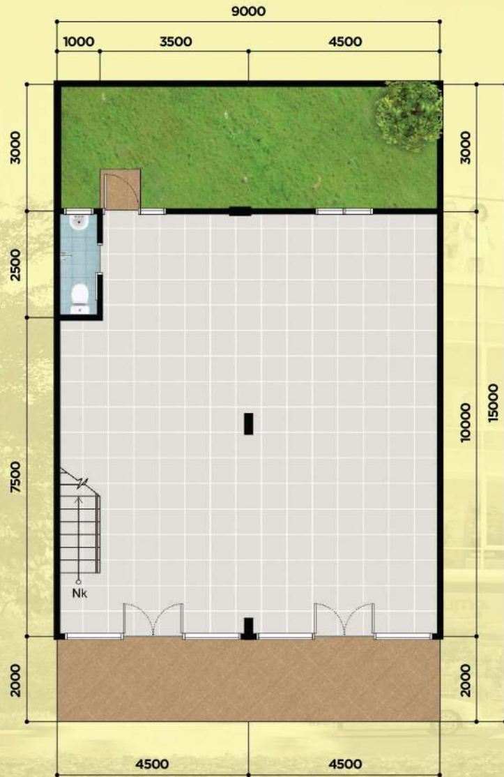
Lantai Dasar
