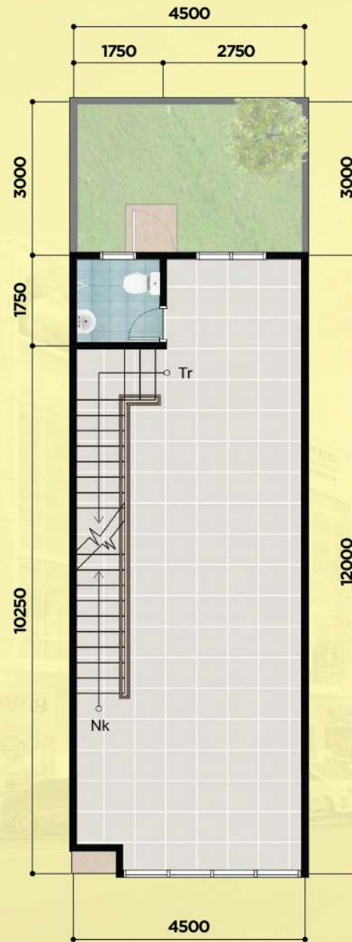
Lantai 2
