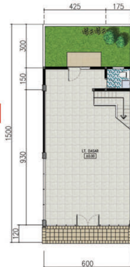
• Denah Lantai 1 •
