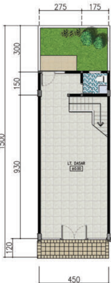
• Denah Lantai 1 •
