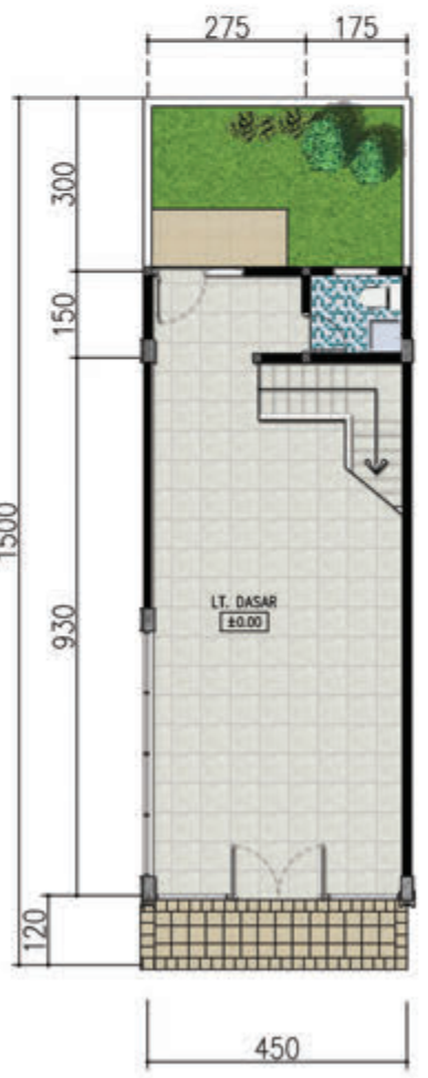
• Denah Lantai 1 •
