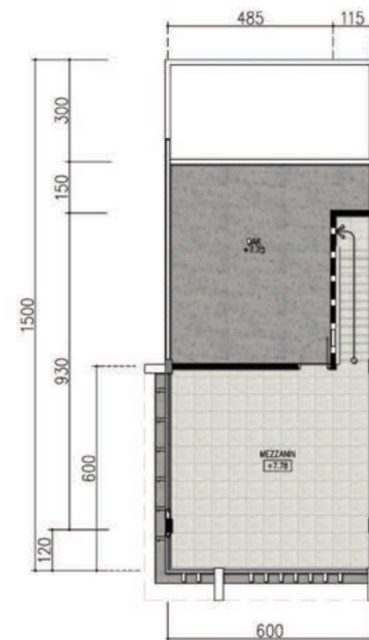
• Denah Lantai 3 •
