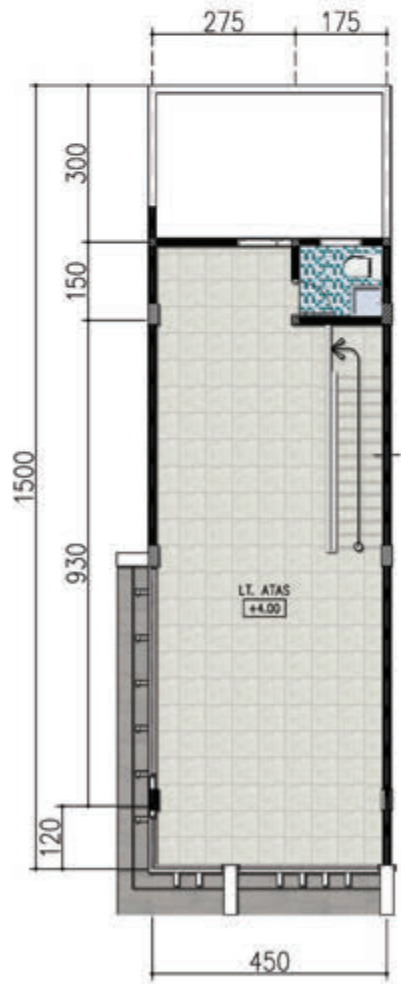
• Denah Lantai 2 •
