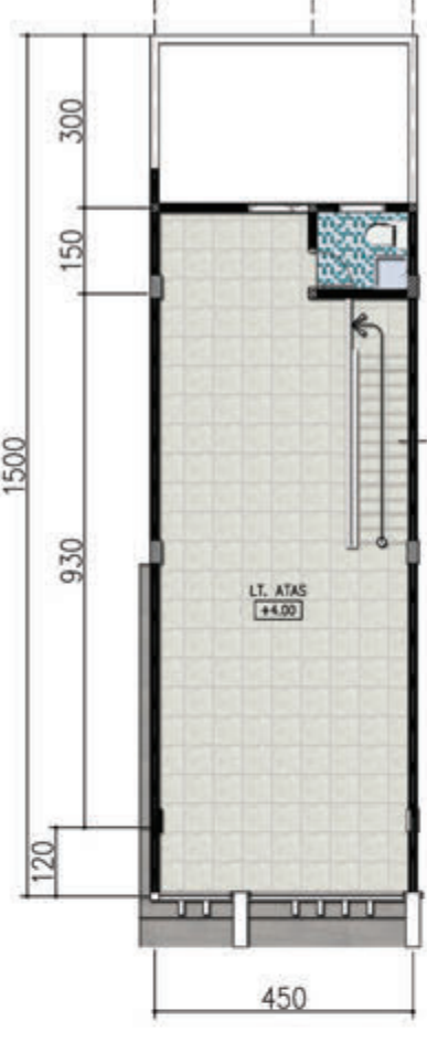
• Denah Lantai 2 •
