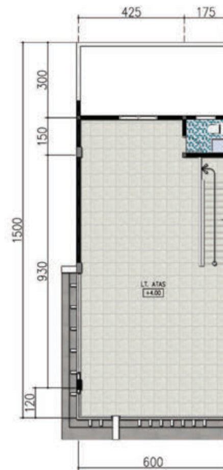
• Denah Lantai 2 •
